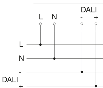
Schema elettrico Master
